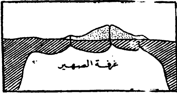
رسم توضيحي بين مصدر اللافا البركانية
